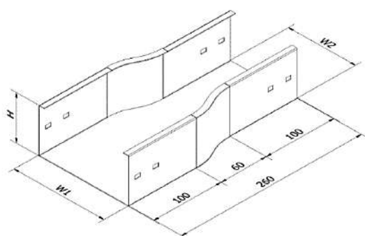
Co giảm W < 200
