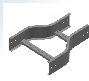
Co Giảm
