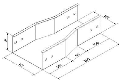
Co giảm W < 200
