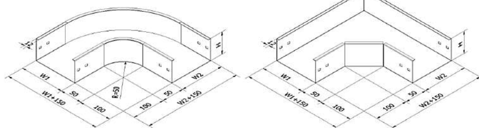
Co ngang W < 200
