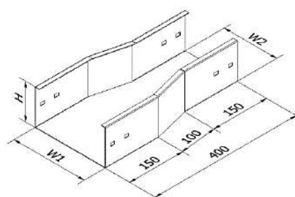
Co giảm W \geq 200
