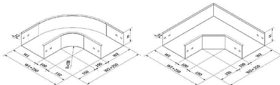
Co ngang W \geq 200
