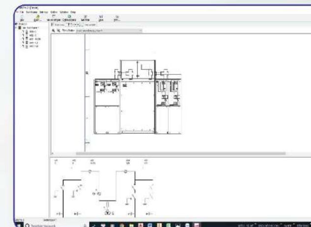
PHẦN MỀM SAFE PRO 3 ABB (CẤU HÌNH TỦ TRUNG THẾ)
